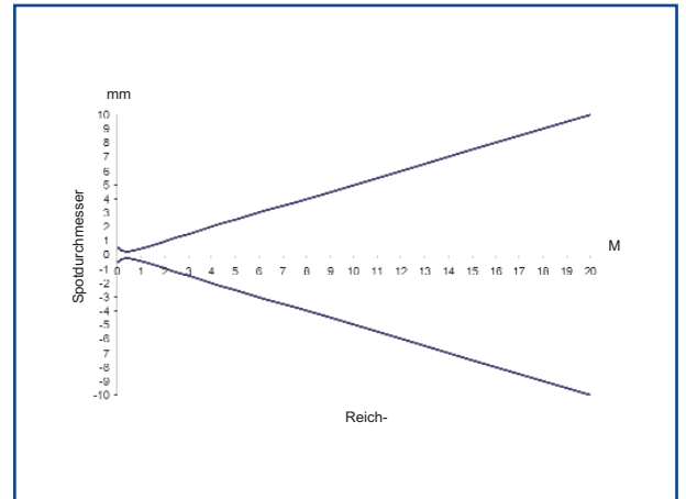
Spotgröße - Polarisierte Laser-Reflexlichtschranke
