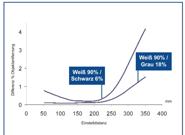
Laser-Hintergrundausbldung 50 ... 350 mm
