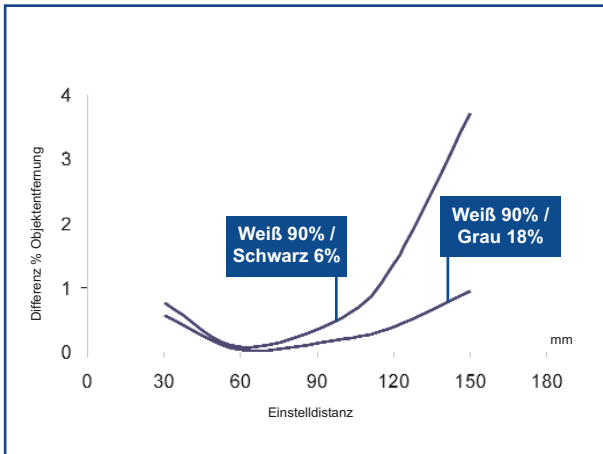
Laser-Hintergrundausbldung 30 ... 150 mm
